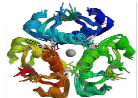
INSULIN-MOLEKÜLE
