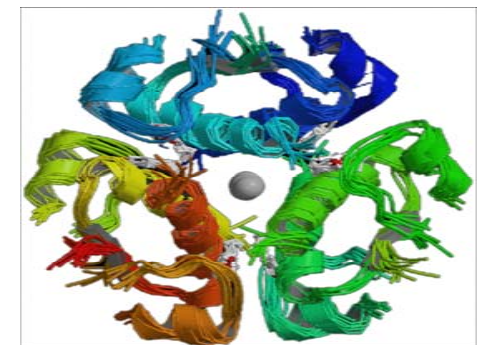
INSULIN-MOLEKÜLE
